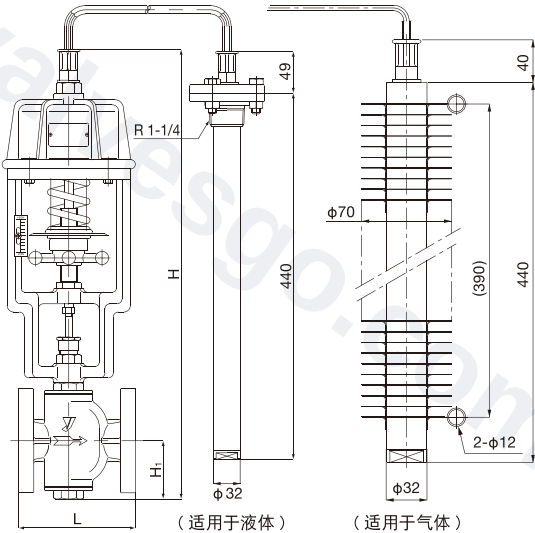
(适用于液体) (适用于气体)
