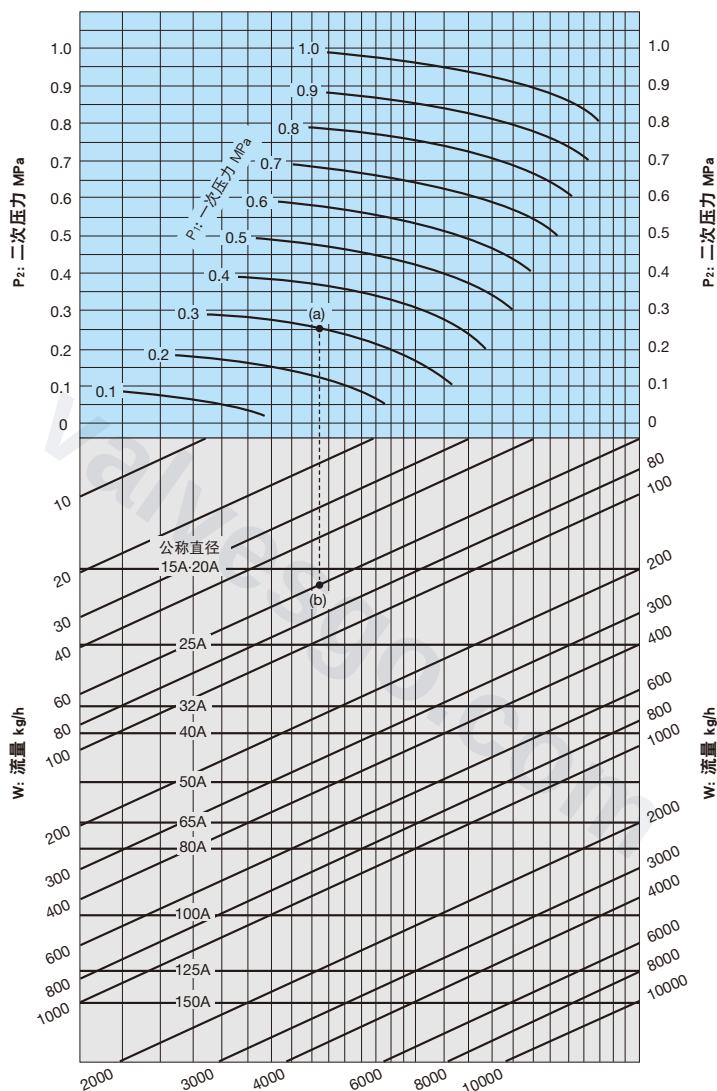
■ 公称直径选择图表 (适用于蒸汽)
