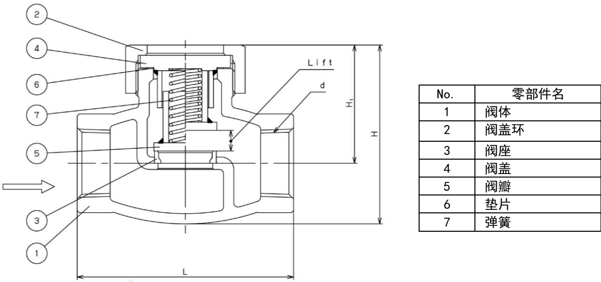
图-1. 構造、尺寸与重量
