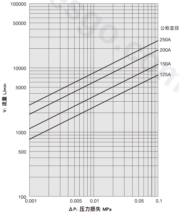
■压力损失图表（适用于水）
