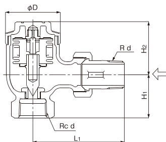
TS-1A (角型)
