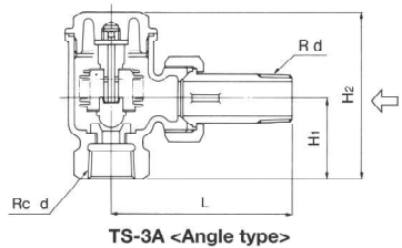
TS-3A <Angle type>
